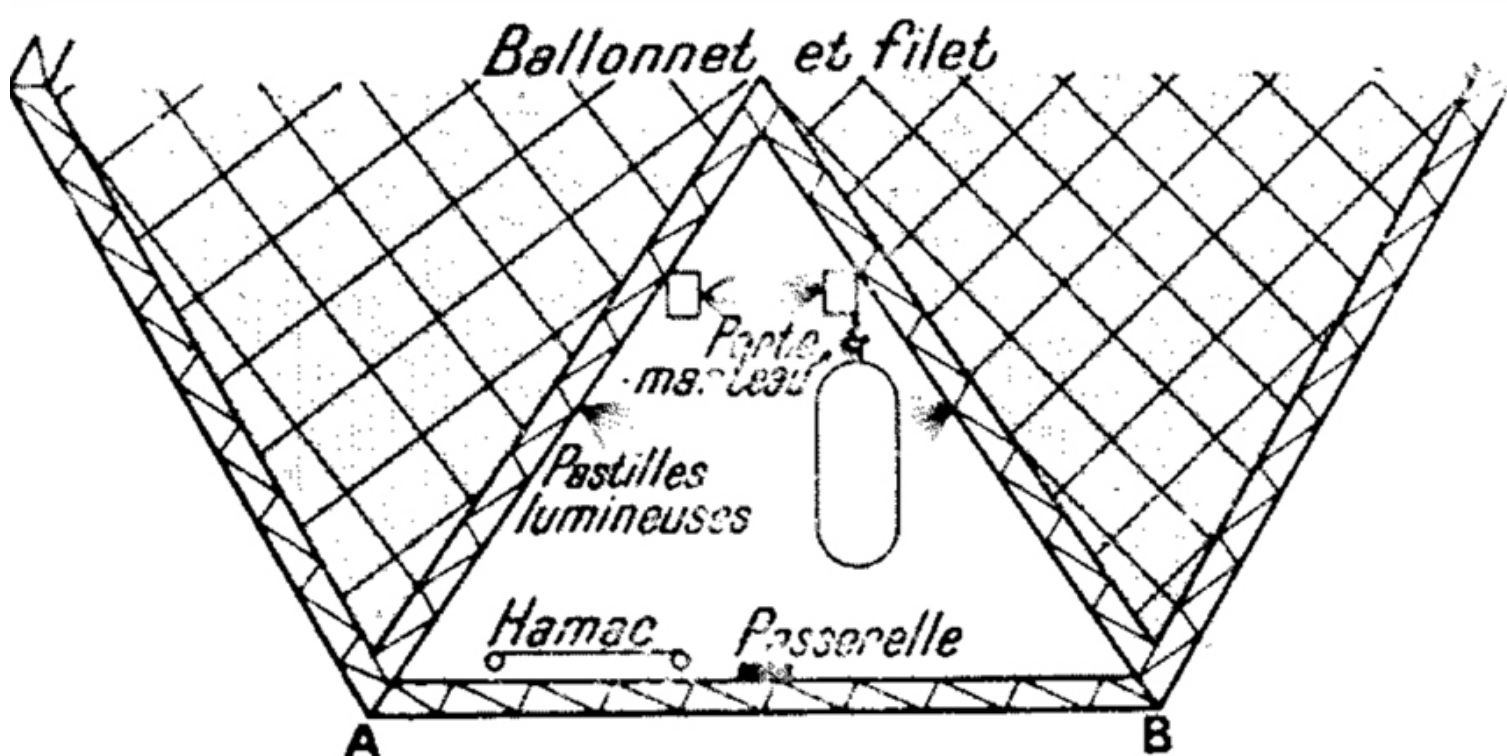
Coupe schématique transversale de la quille : en réalité les réservoirs d'essence, bombes, water-ballast sont accrochés face à face par groupes de deux aux portemanteaux.
