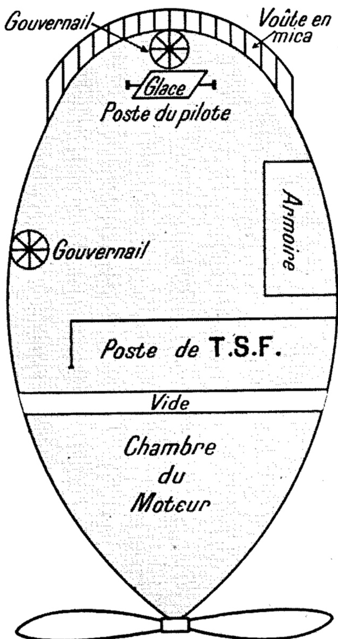
Plan schématique de la nacelle avant.
