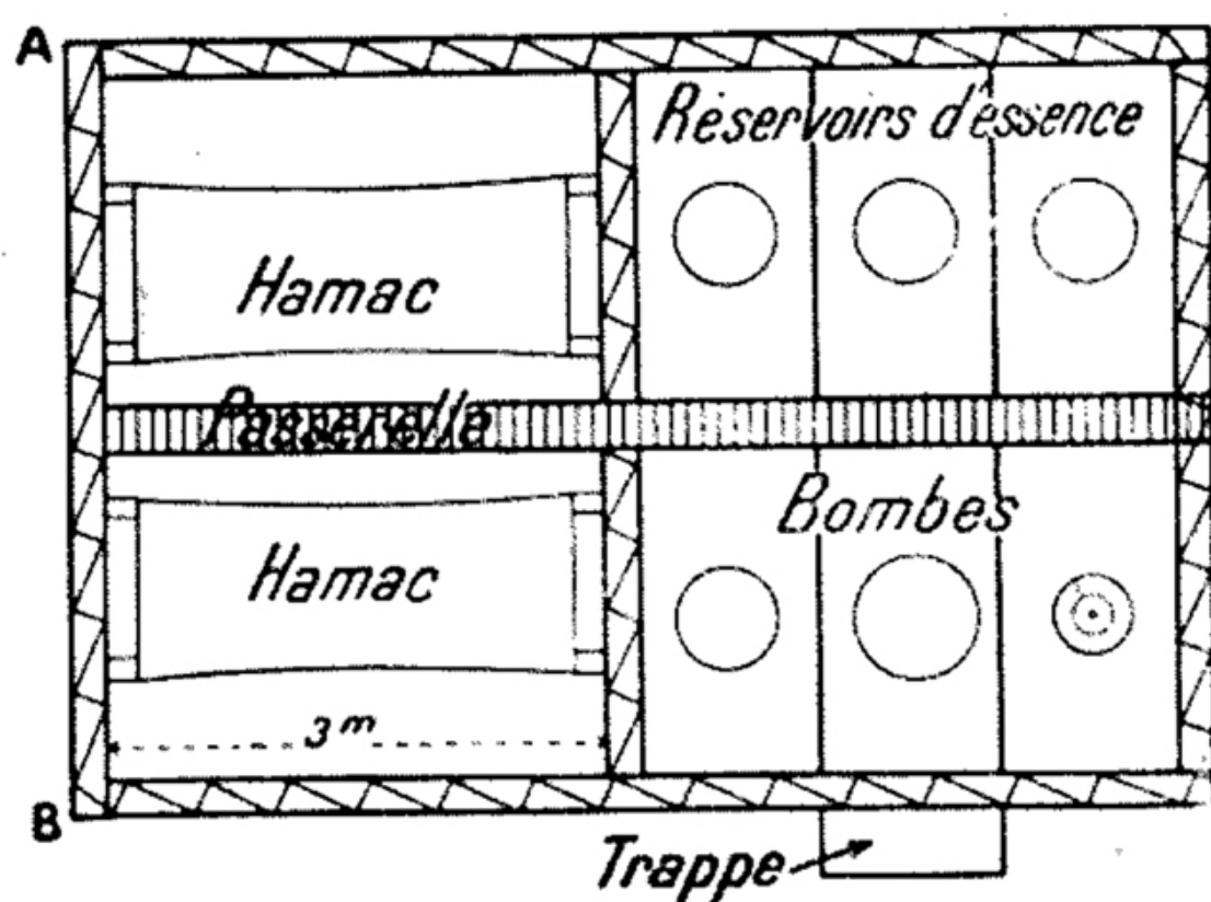
Plan schématique longitudinal d'un des panneaux formant le plancher de la quille.
